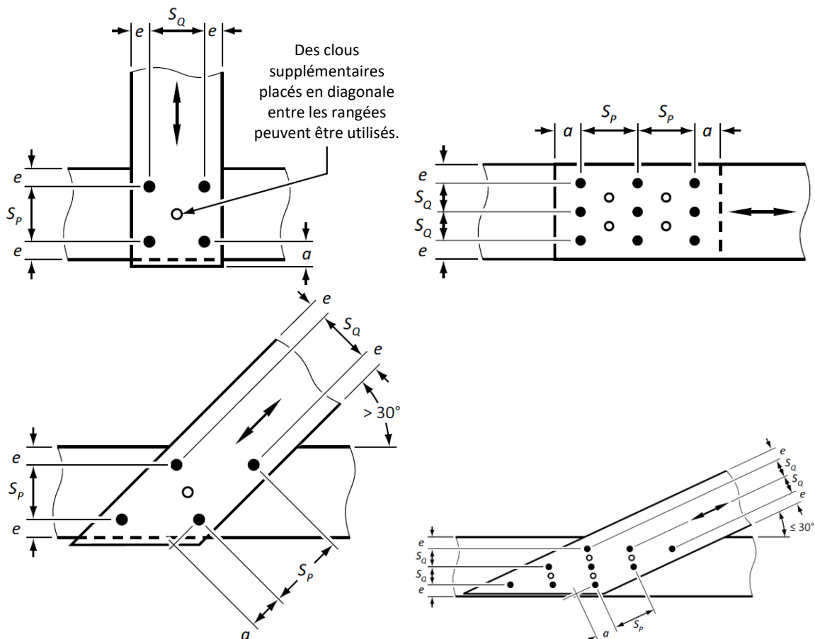
Figure 2. Exemple de schémas qui indiquent l'espacement de la fixation 14
